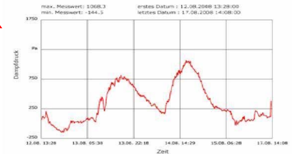
Dampfdruck Differenz Dach BT2 - Aussen
